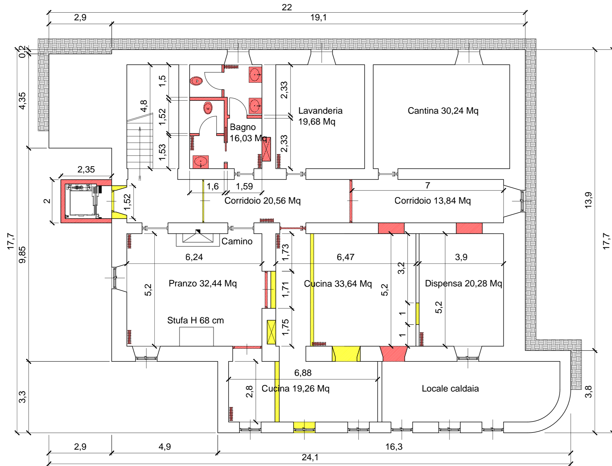
PIANTA PIANO INTERRATO - STATO DI PROGETTO
